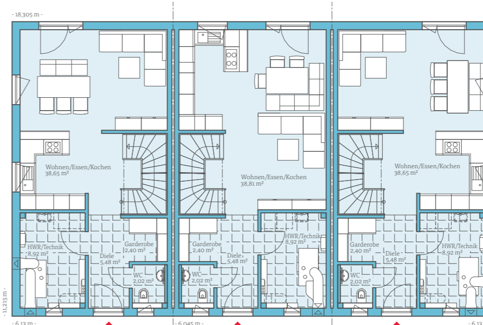
ERDGESCHOSS
