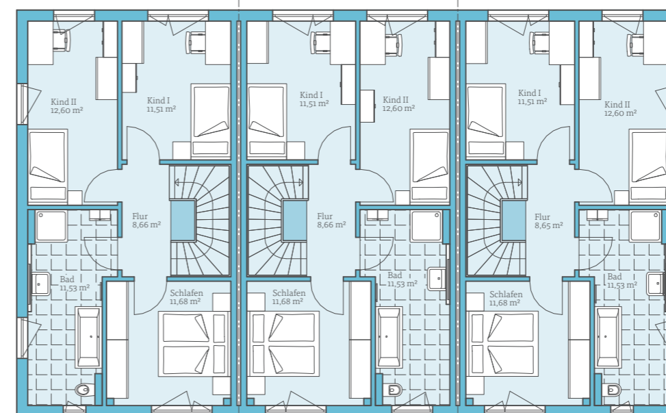
OBERGESCHOSS
