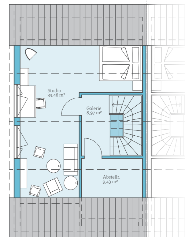
DACHGESCHOSS
