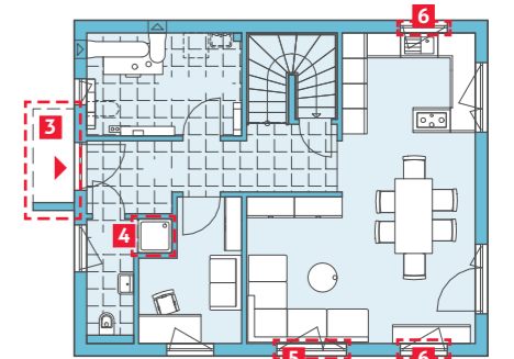
ERDGESCHOSS
