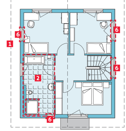
OBERGESCH.
