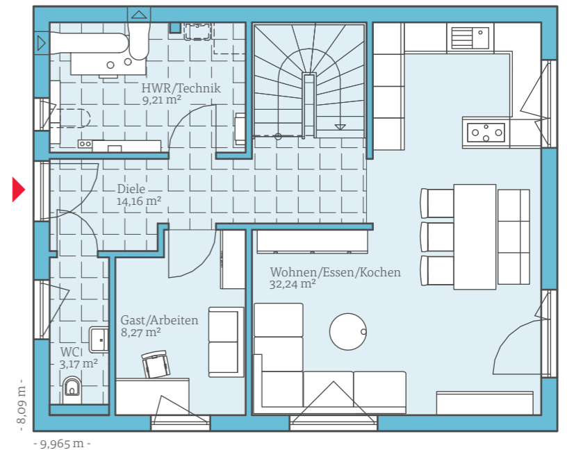
ERDGESCHOSS
